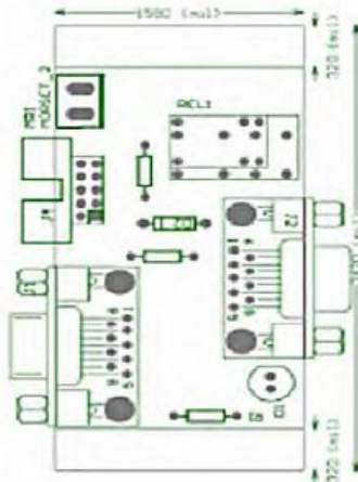
Schema dei collegamenti dello schedino deviatore:
